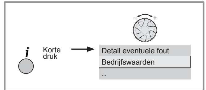
figuur 11 - Informatietoets
