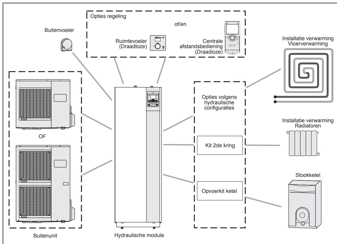
figuur 1 - Overzicht van een volledige configuratie van een installatie
