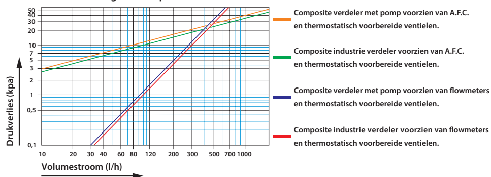
Drukverliesdiagramm composite verdelers
